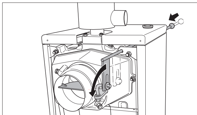
Rys. 25 Otwarcie klapy odcinającej przepływ spalin
