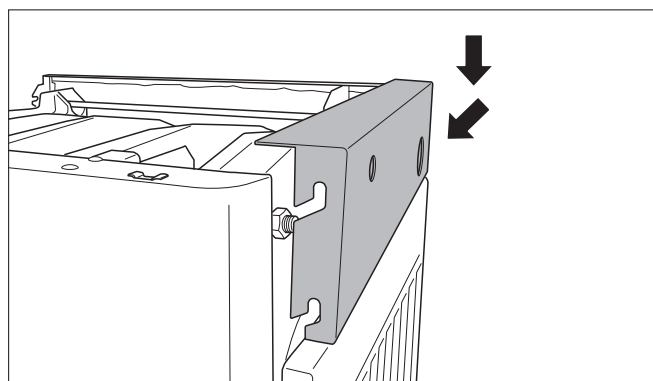
Rys. 8 Montaż blachy frontowej
