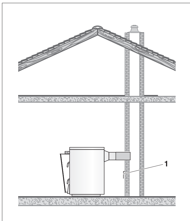
Rys. 13 Przyłączenie do instalacji odprowadzania spalin
