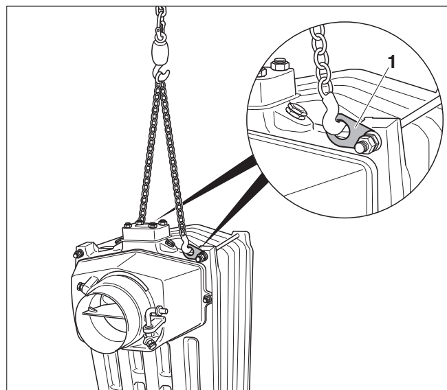
Rys. 5 Transport kotła grzewczego przy użyciu dźwigu
