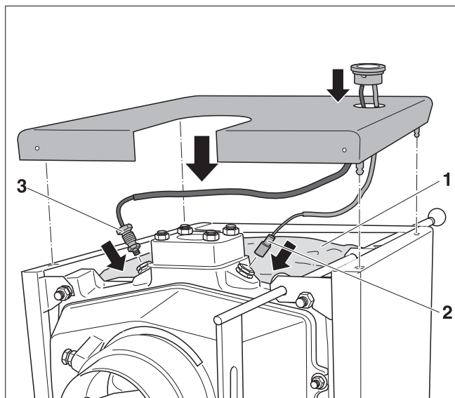
Rys. 10 Montaż pokrywy kotła i termomanometru
