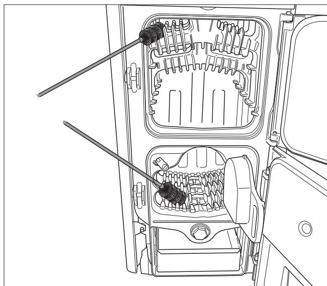
Rys. 26 Czyszczenie kanałów przepływu spalin
