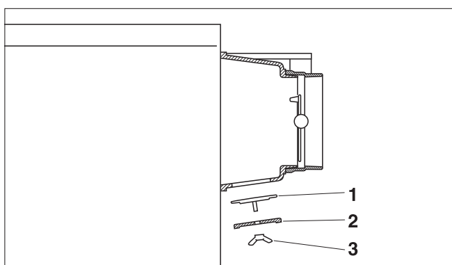
Rys. 27 Pokrywa wyczystki na króćcu rury spalinowej.
