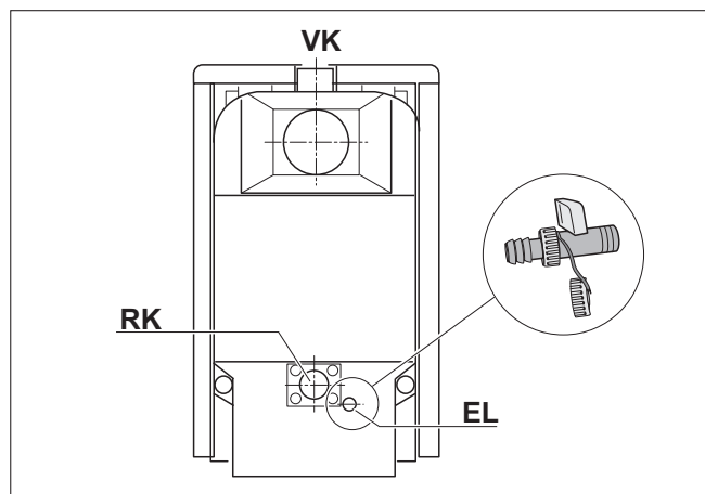
Rys. 14 Wykonanie przyłączy hydraulicznych
