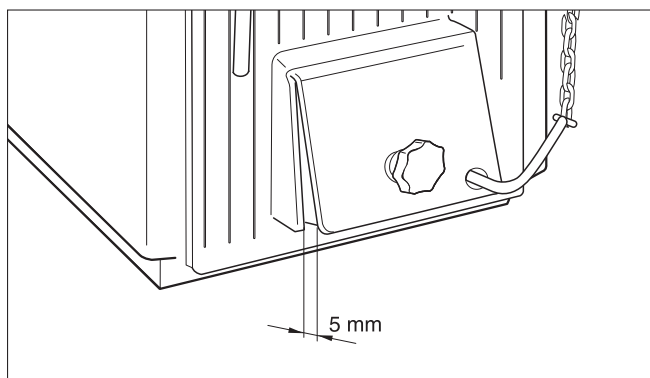
Rys. 22 Ustawienie otwarcia kłapy powietrza
