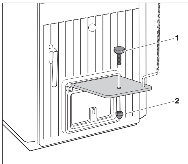
Rys. 12 Przymocowanie łańcucha do klapy powietrza
