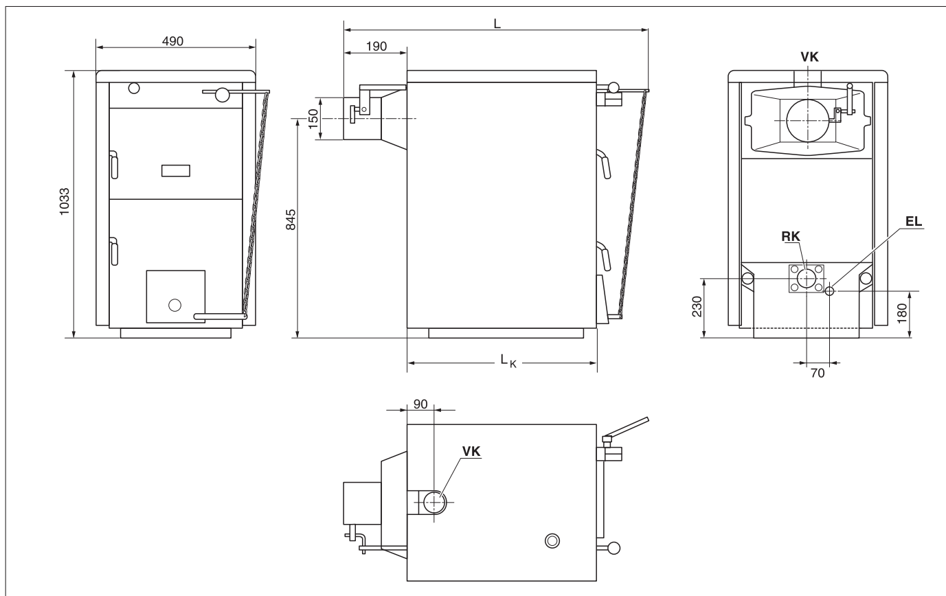
Rys. 2 Wymiary i przyłącza (wymiary w mm)
