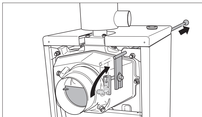
Rys. 21 Zamknięcie kłapy odcinającej przepływ spalin
