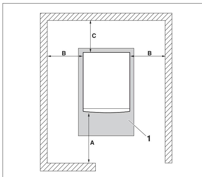
Rys. 6 Odstępy od ścian w kotłowni
