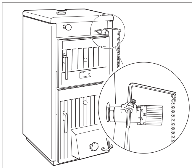
Rys. 18 Ustawienie napięcia łańcucha
