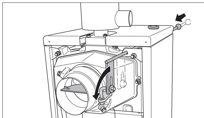
Rys. 20 Otwarcie kłapy odcinającej przepływ spalin
